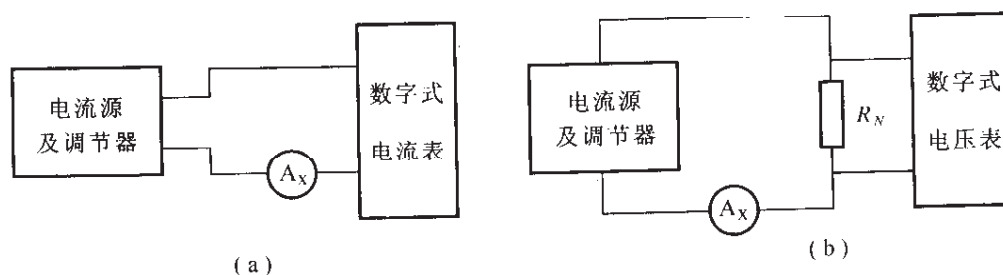
图 1 用数字表检定电流表的接线图
