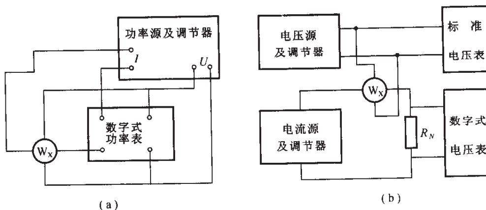
图3 用数字表检定功率表的接线图
