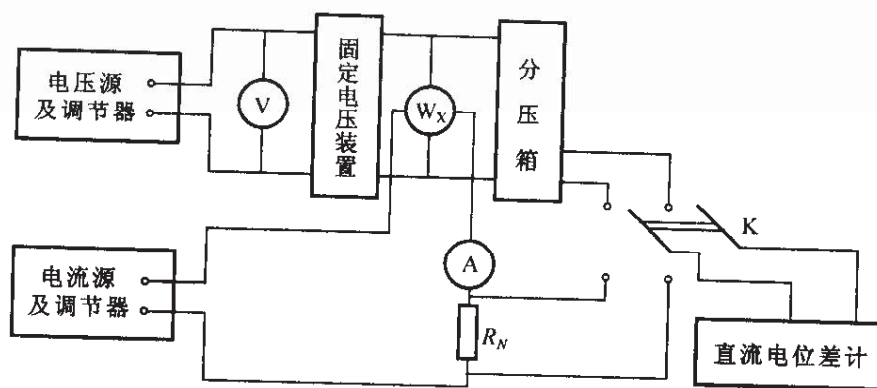
图 10 检定直流功率表的接线图
