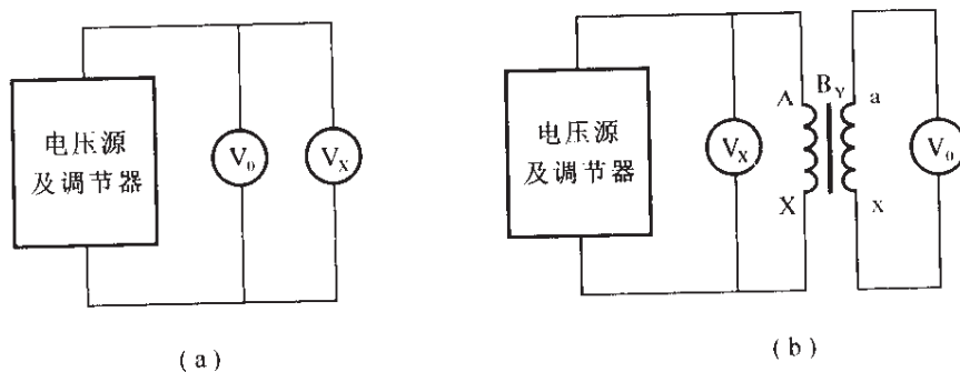
图5 检定电压表接线图
