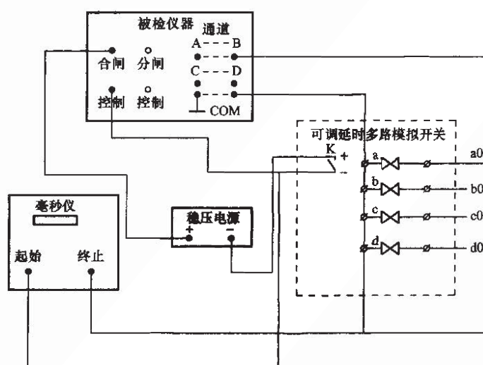
图 1 合闸时间测量
