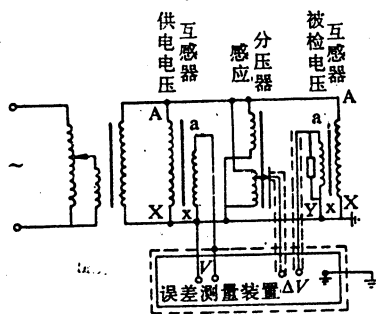
图5 比较线路（高电位端测量误差）
