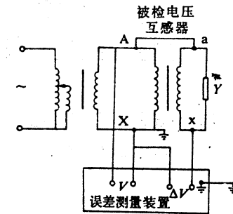
图2 自检线路（低电位端测量误差）
