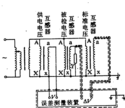
图3 比较线路（高电位端测量误差）
