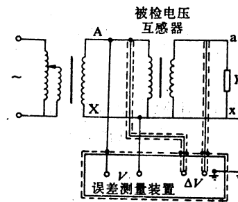
图1 自检线路（高电位端测量误差）
