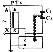
图 3 阻抗电桥型
