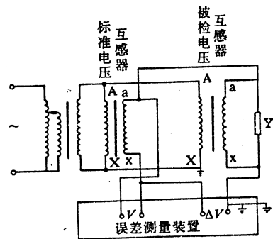
图4 比较线路（低电位端测量误差）
