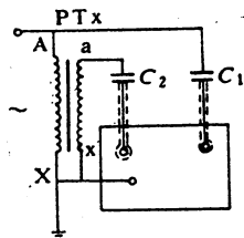
图 1 电流比较仪电桥型
