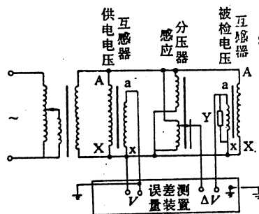
图6 比较线路（低电位端测量误差）
