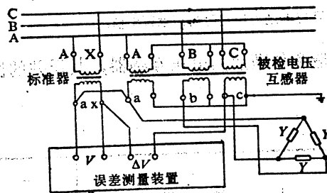
图7 三相电压互感器检定线路
