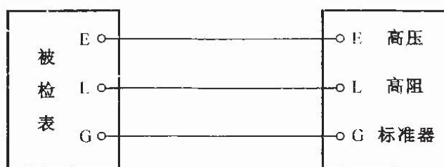
图 1 示值误差检定接线图
